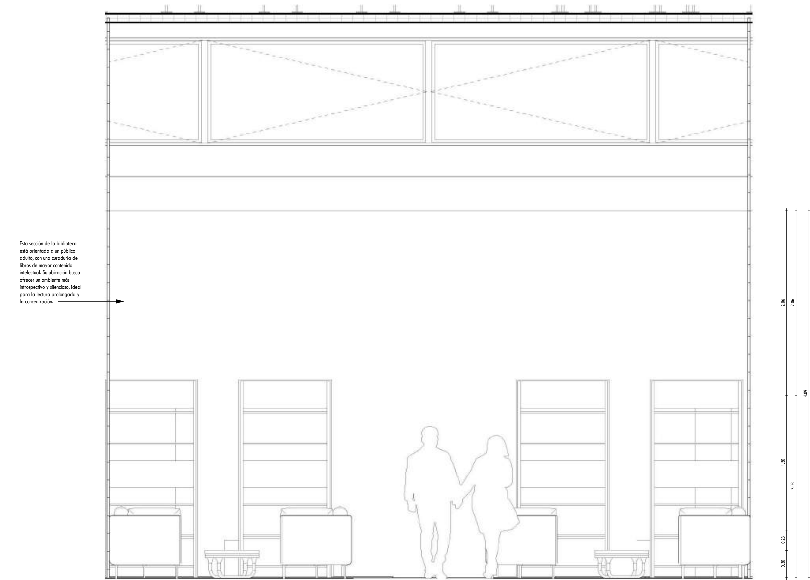
1 DE - ELEVACION LONGITUDINAL AA AREA DE LECTURA A-39 1 : 25
