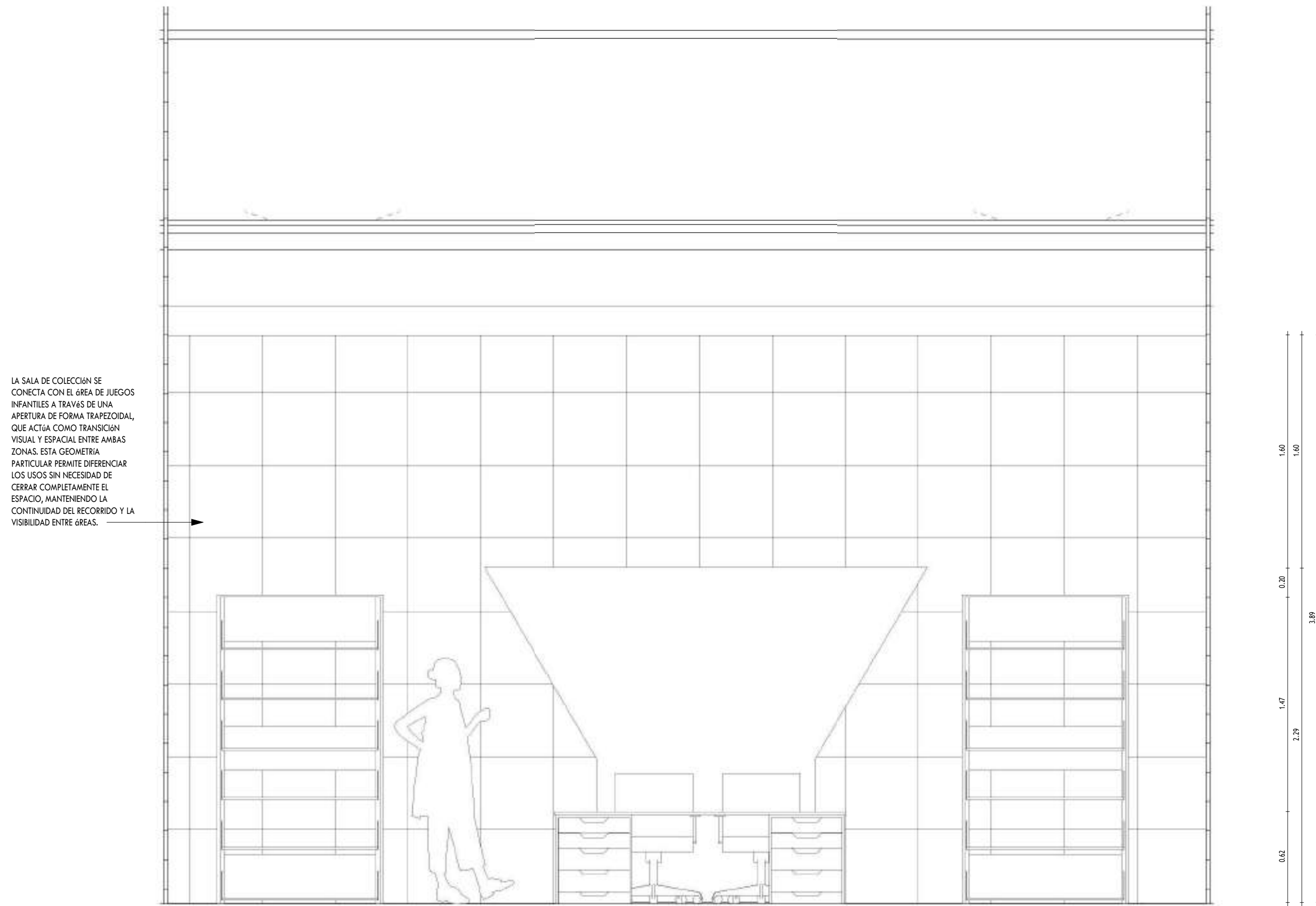
2 DE - ELEVACION LONGITUDINAL AA SALA DE COLECCION 1 : 25 0 .5m
