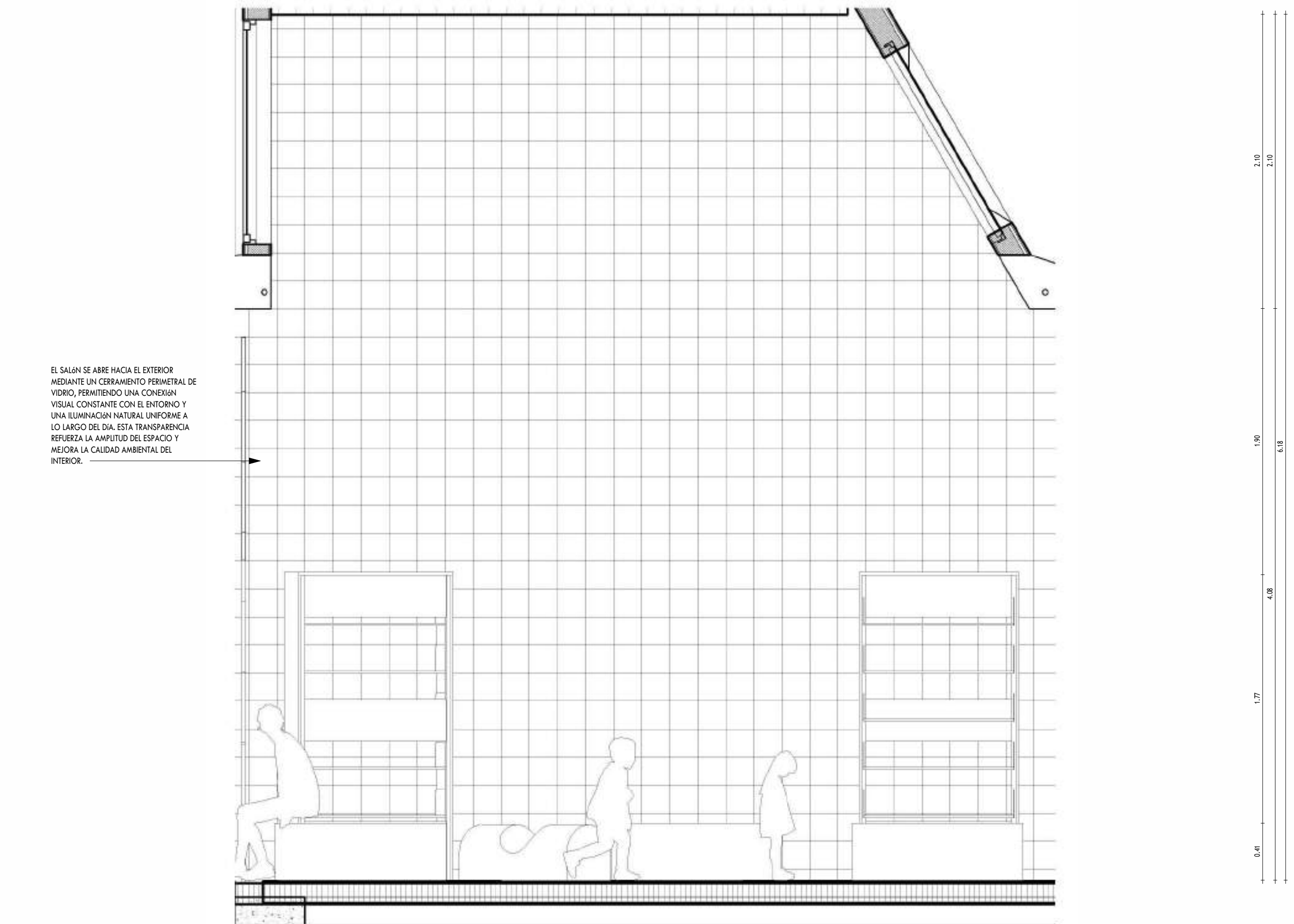
2 DE - ELEVACION TRANSVERSAL AA SALA INFANTIL A-38 1 : 25
