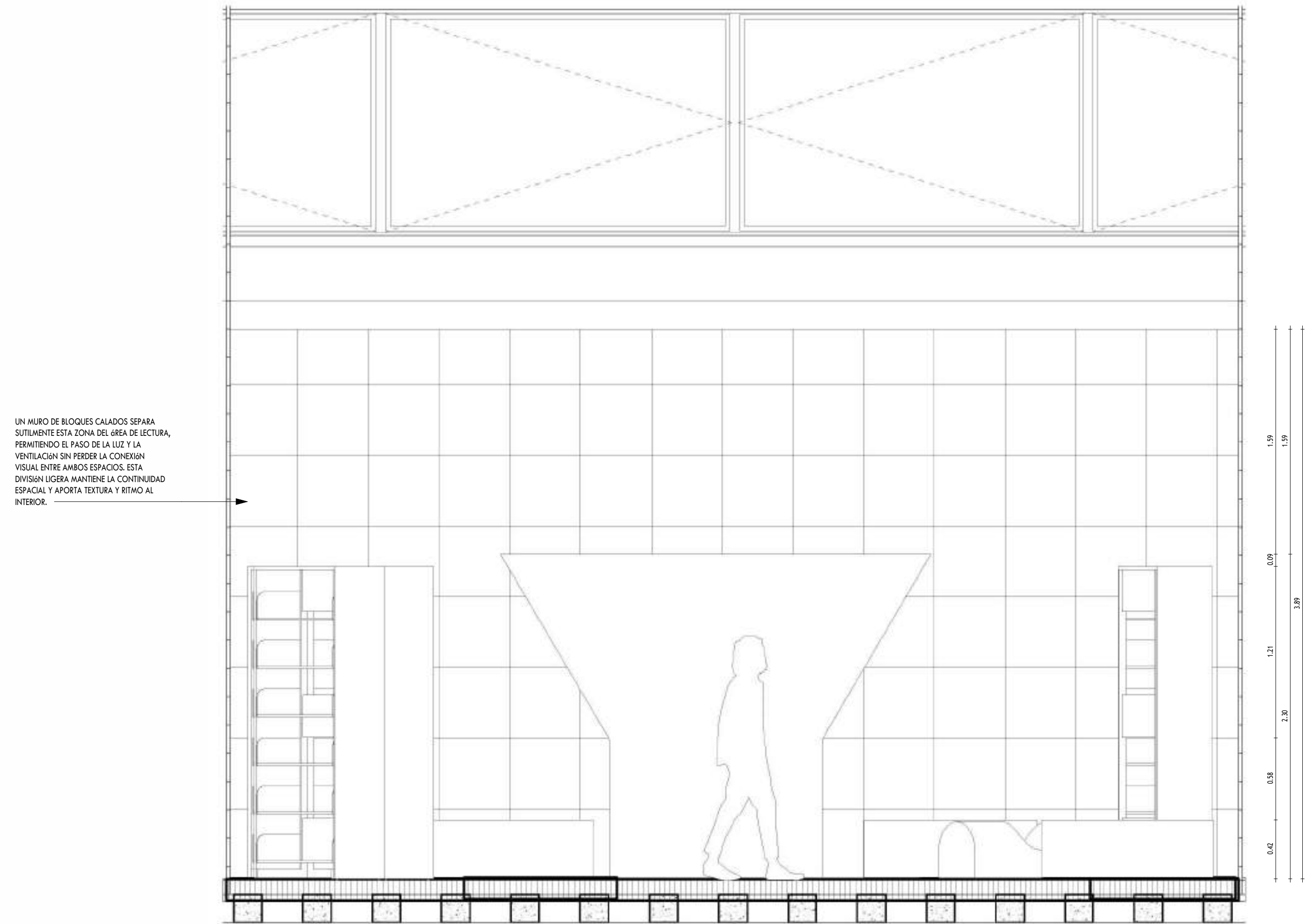
1 DE - ELEVACION LONGITUDINAL AA SALA INFANTIL A-38 1 : 25
