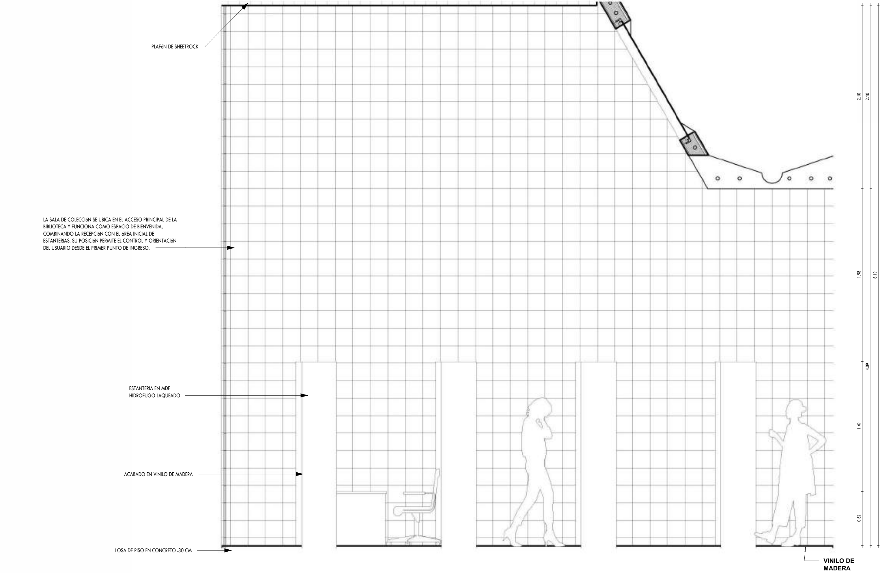
1A DE - ELEVACION TRANSVERSAL AA SALA DE COLECCION 1 : 25 0 .5m
