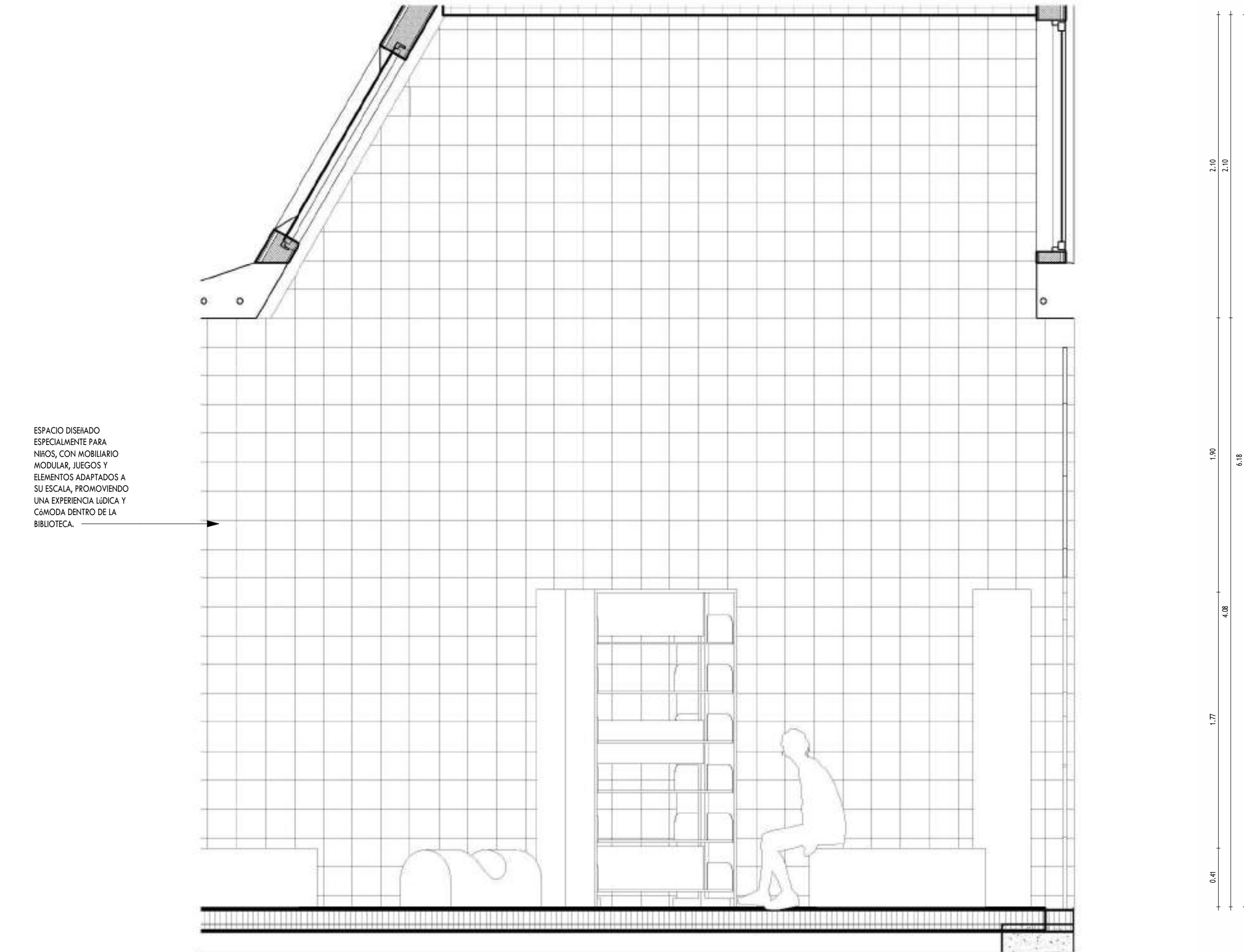
4 DE - ELEVACION TRANSVERSAL BB SALA INFANTIL A-38 1 : 25
