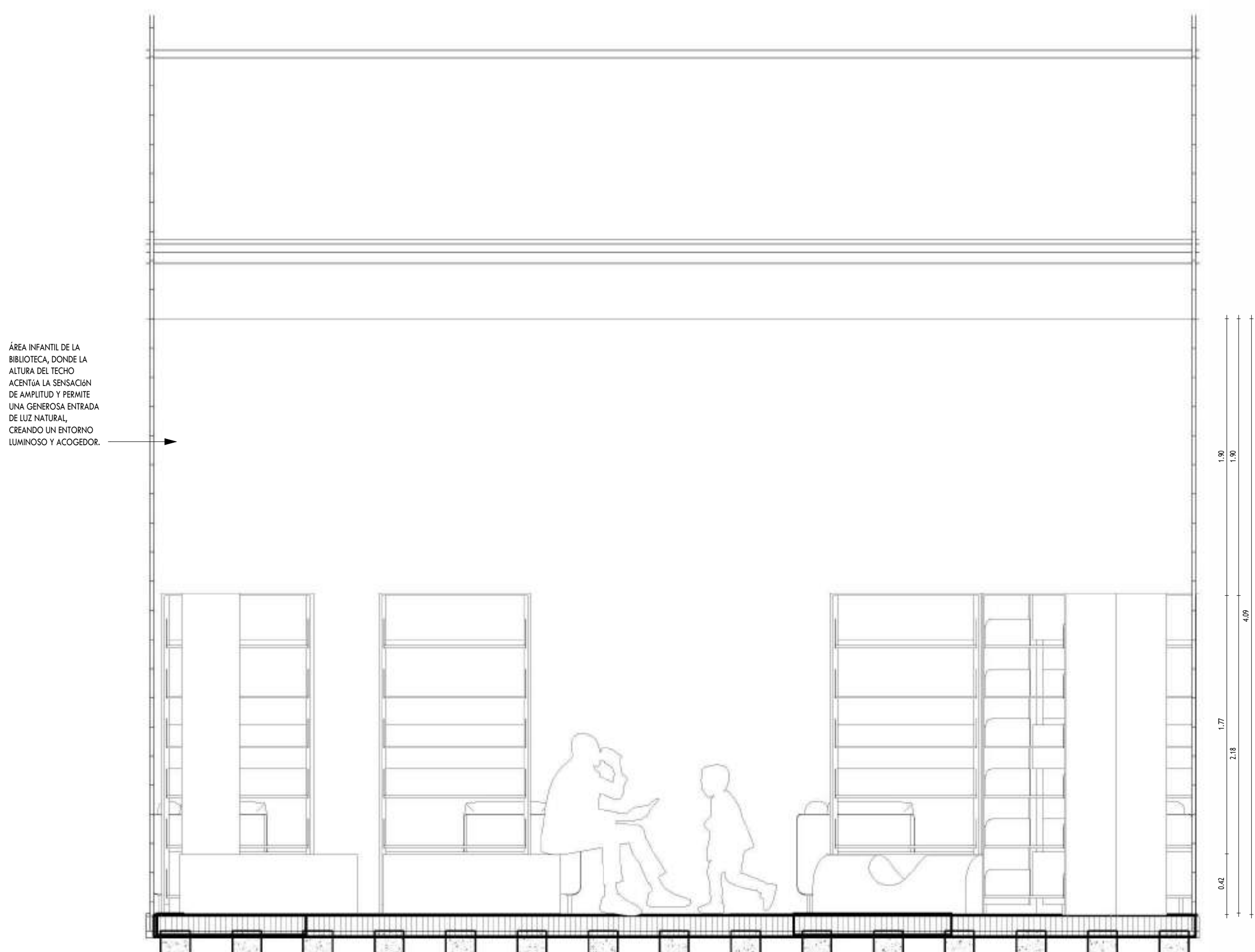
3 DE - ELEVACION LONGITUDINAL BB SALA INFANTIL A-38 1 : 25
