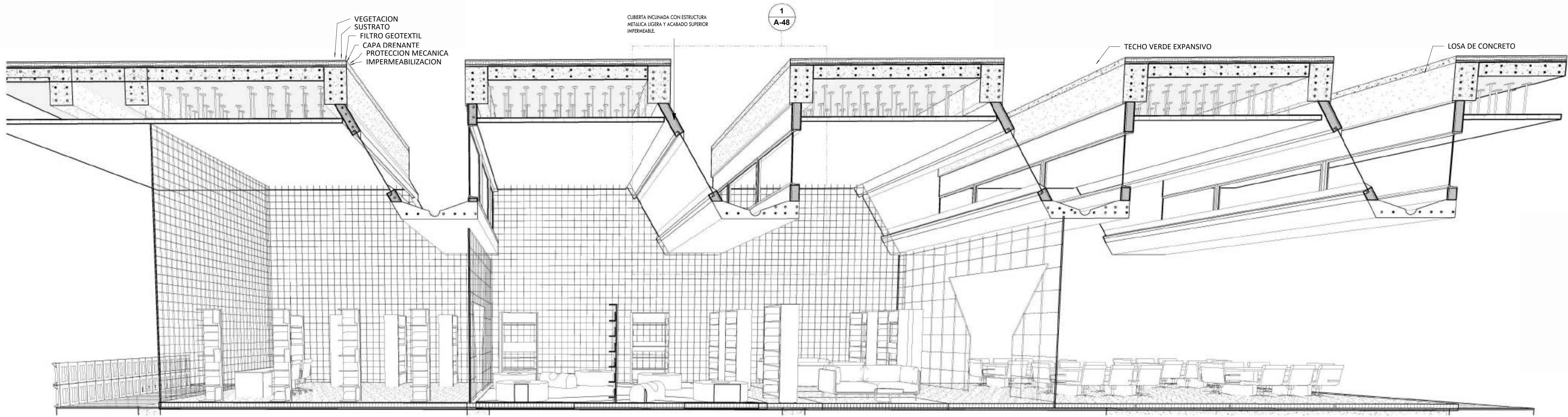
1 A-43 SECCION FUGADA LONGITUDINAL AA
