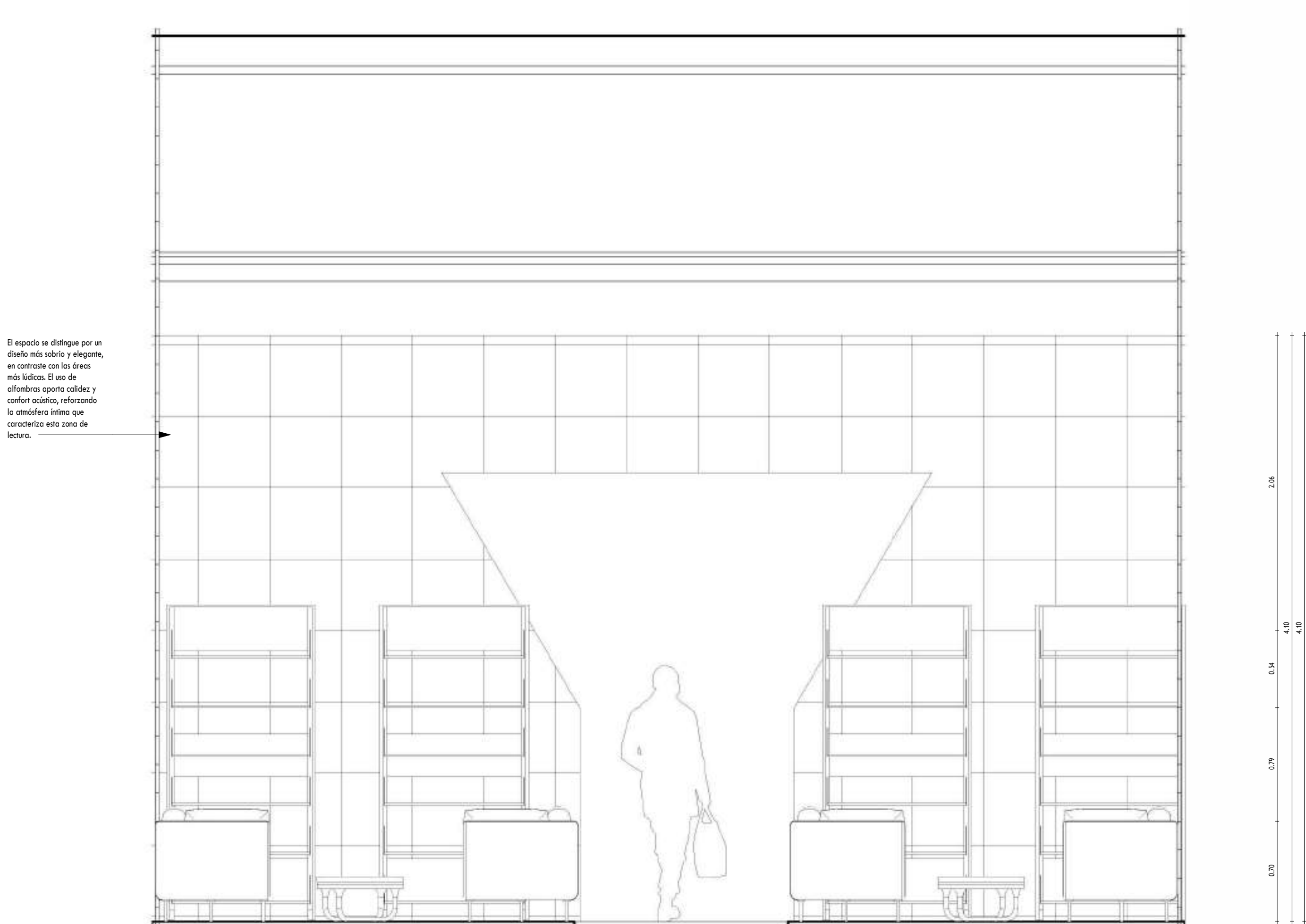
3 DE - ELEVACION LONGITUDINAL BB AREA DE LECTURA A-39 1 : 25
