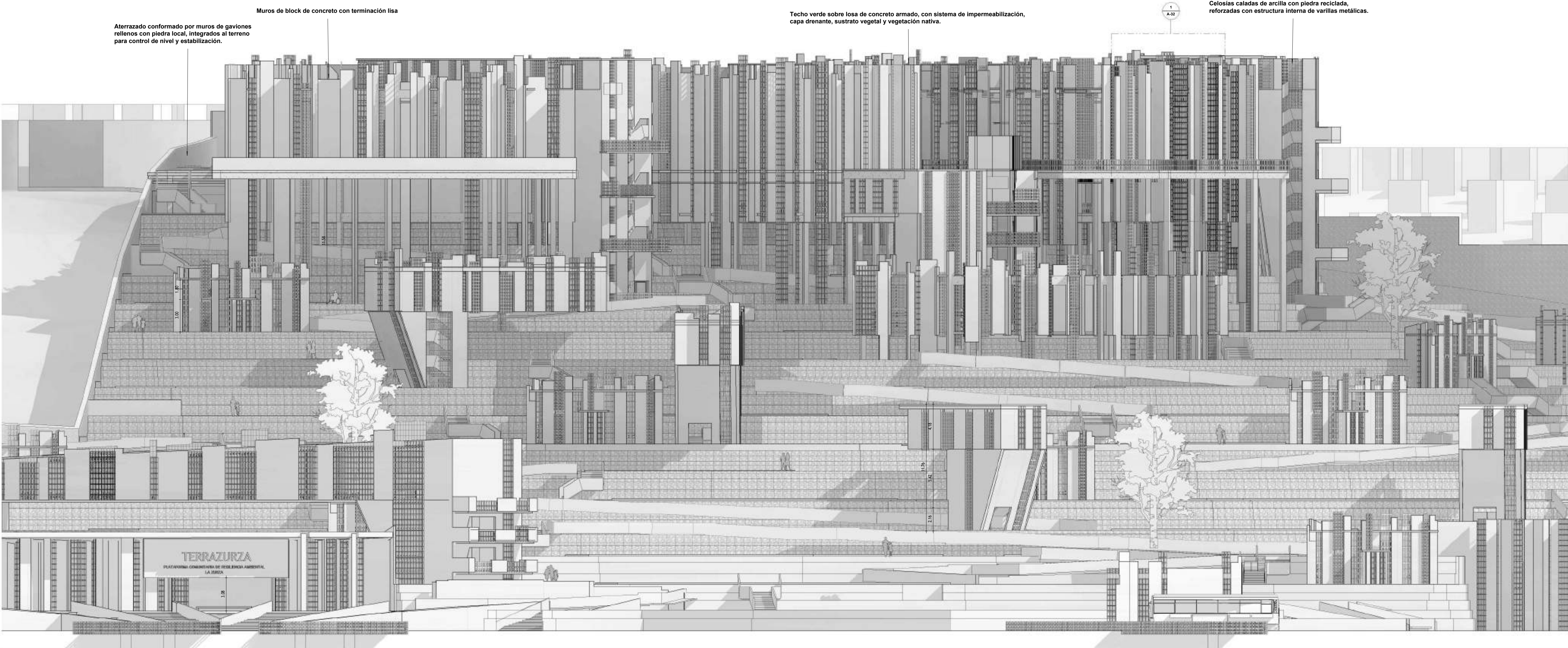
2 A-25 ELEVACION SUR PLATAFORMA COMUNITARIA 1 : 200 0 1 2 3 4 5 10m
