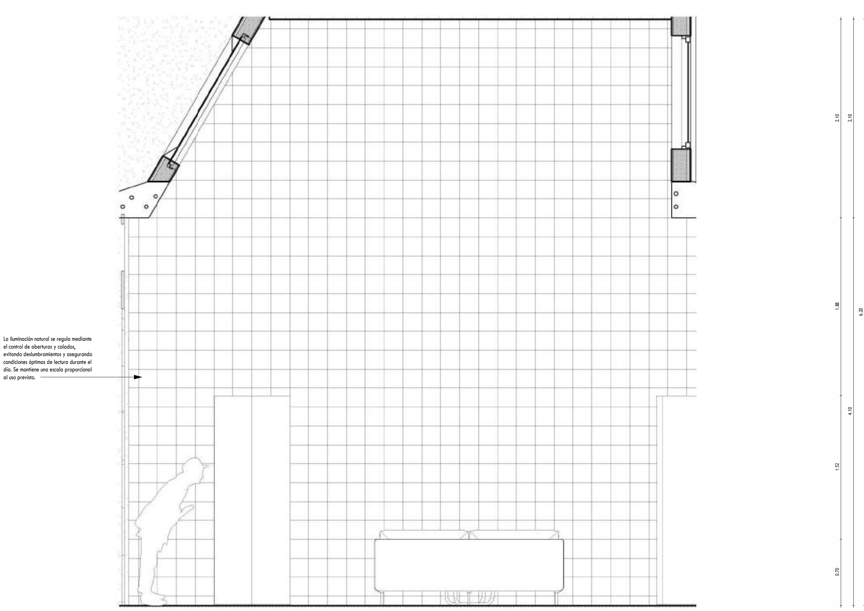
4 DE - ELEVACION TRANSVERSAL BB AREA DE LECTURA A-39 1 : 25
