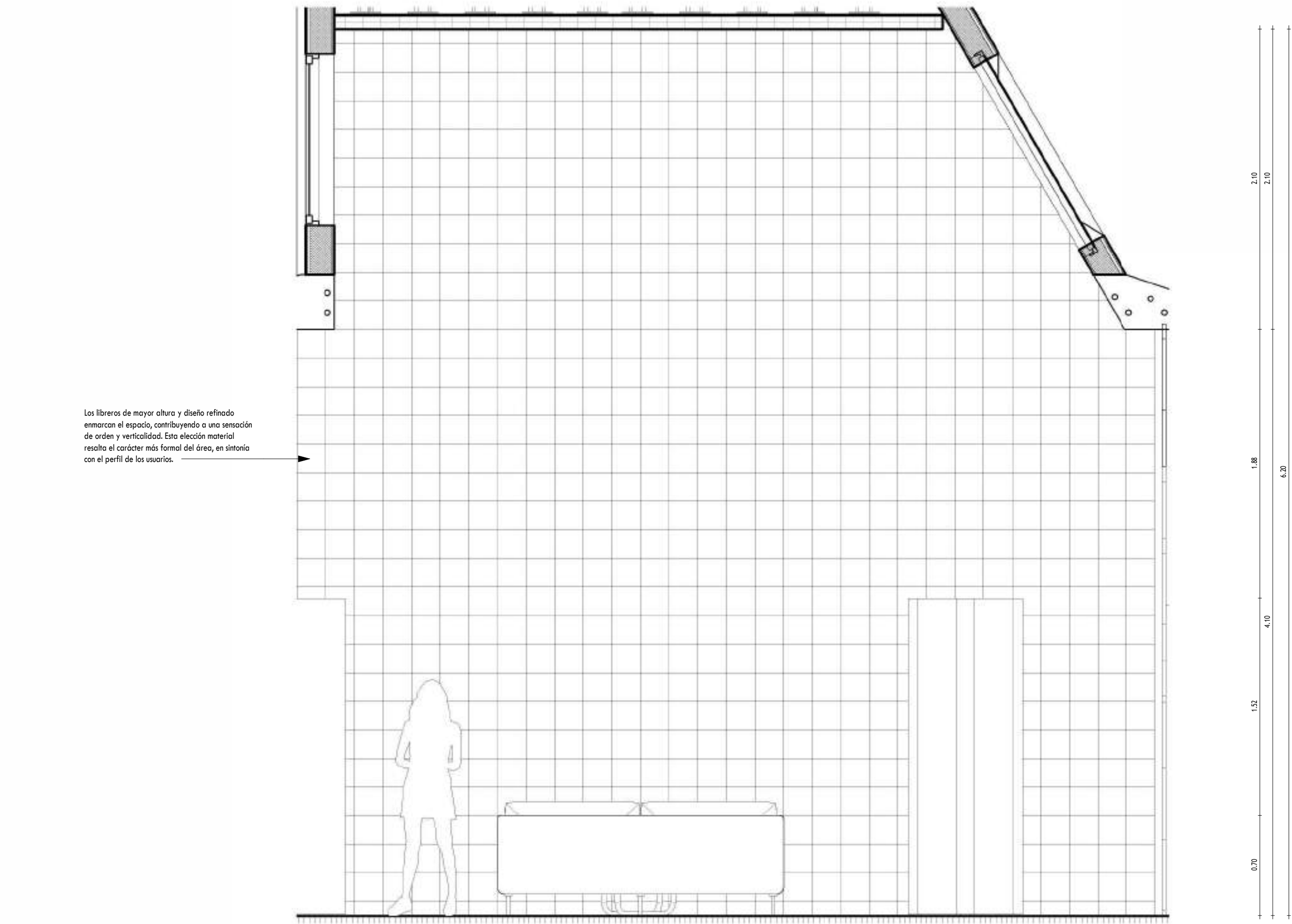
2 DE - ELEVACION TRANSVERSAL AA AREA DE LECTURA A-39 1 : 25
