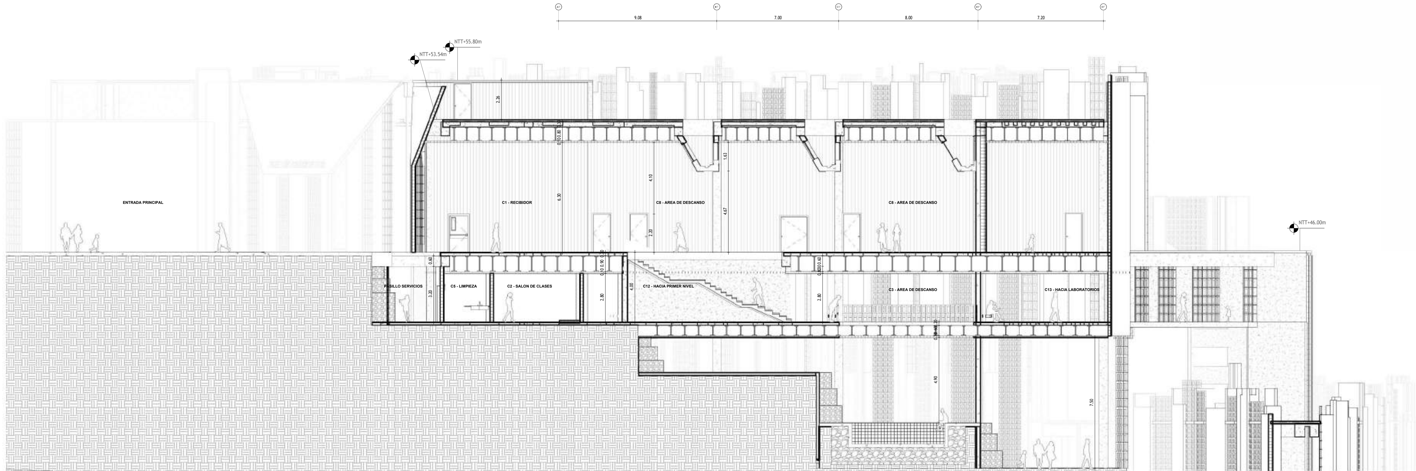
1 SECCION EE - ACERCAMIENTO AULAS DE CLASE 1 : 125
