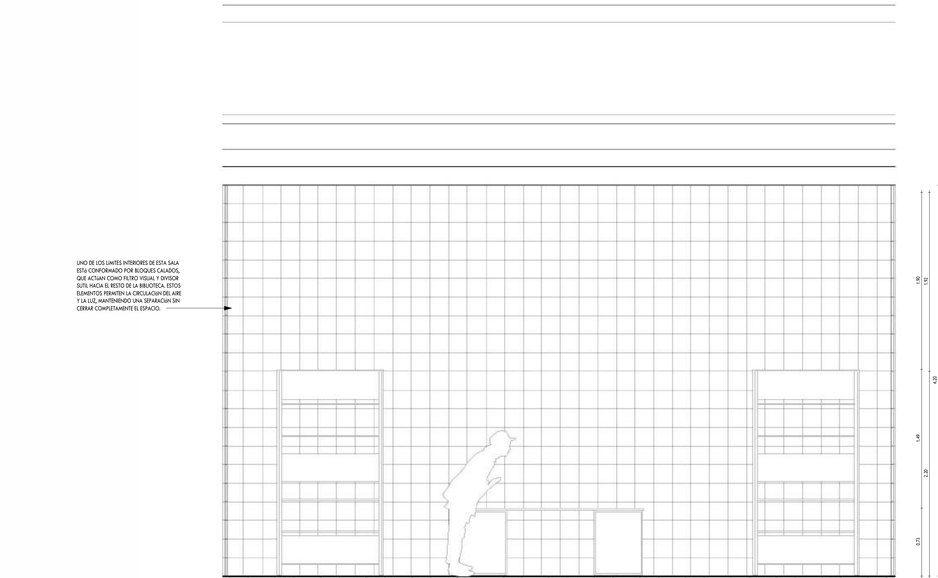
1 DE - ELEVACION LONGITUDINAL BB SALA DE COLECCION 1 : 25 0 .5m
