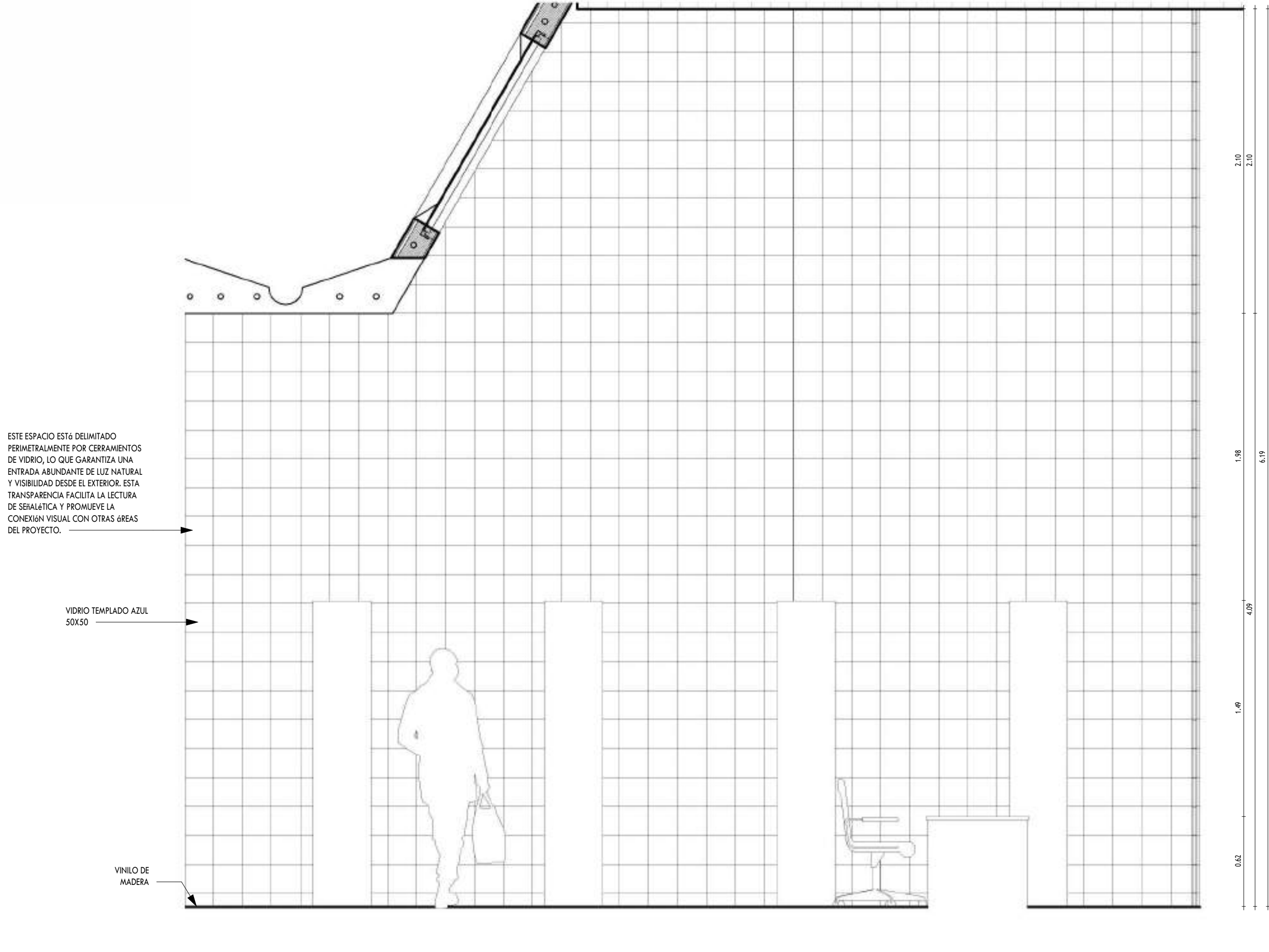
2B DE - ELEVACION TRANSVERSAL BB SALA DE COLECCION 1 : 25 0 .5m
