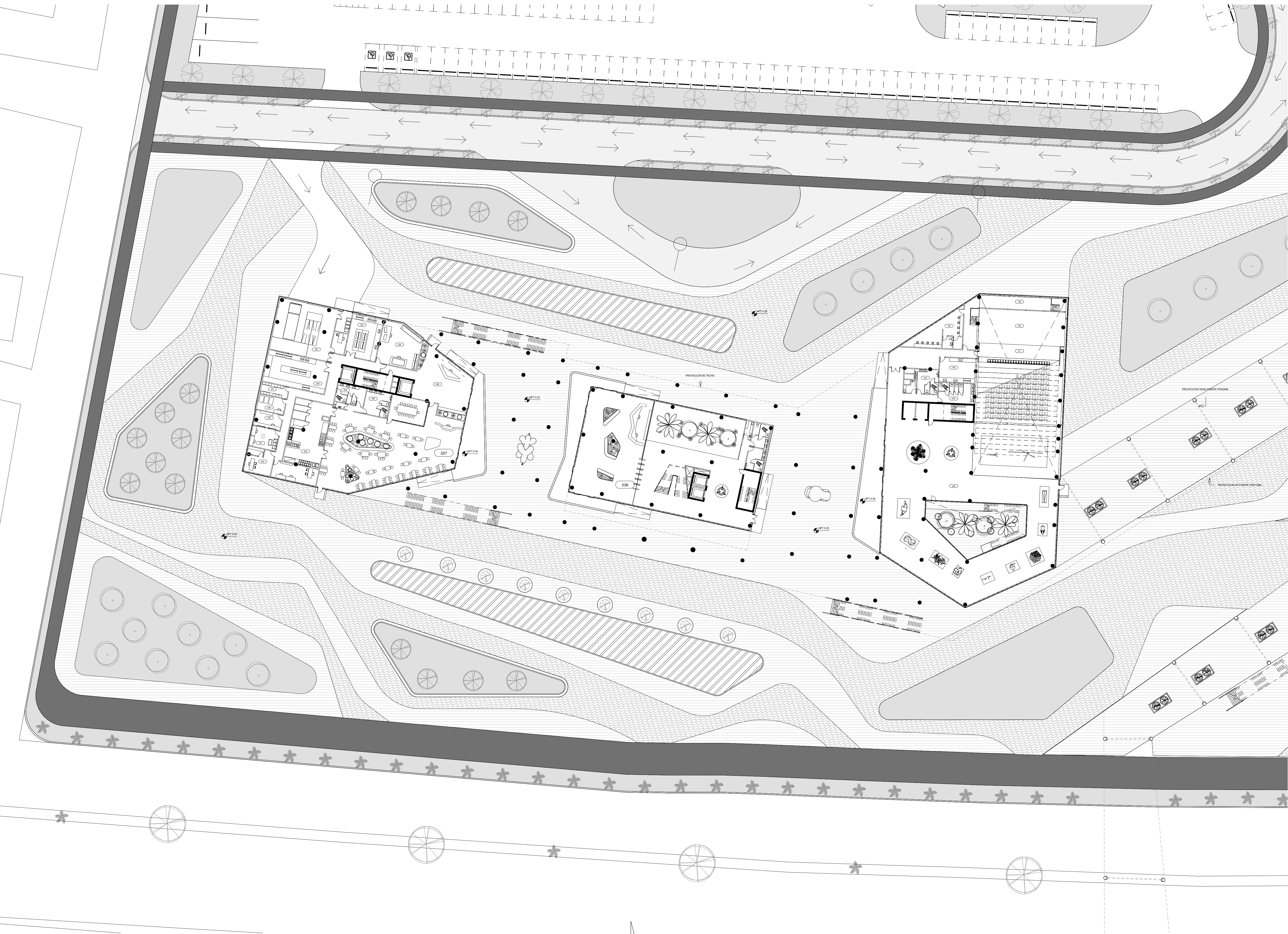
1 G-07 PLANTA ARQUITECTÓNICA AMUEBLADA ZONA C-E 1 : 350
