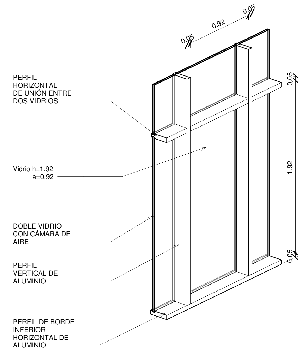
3 DETALLE MURO CORTINA 1:20
