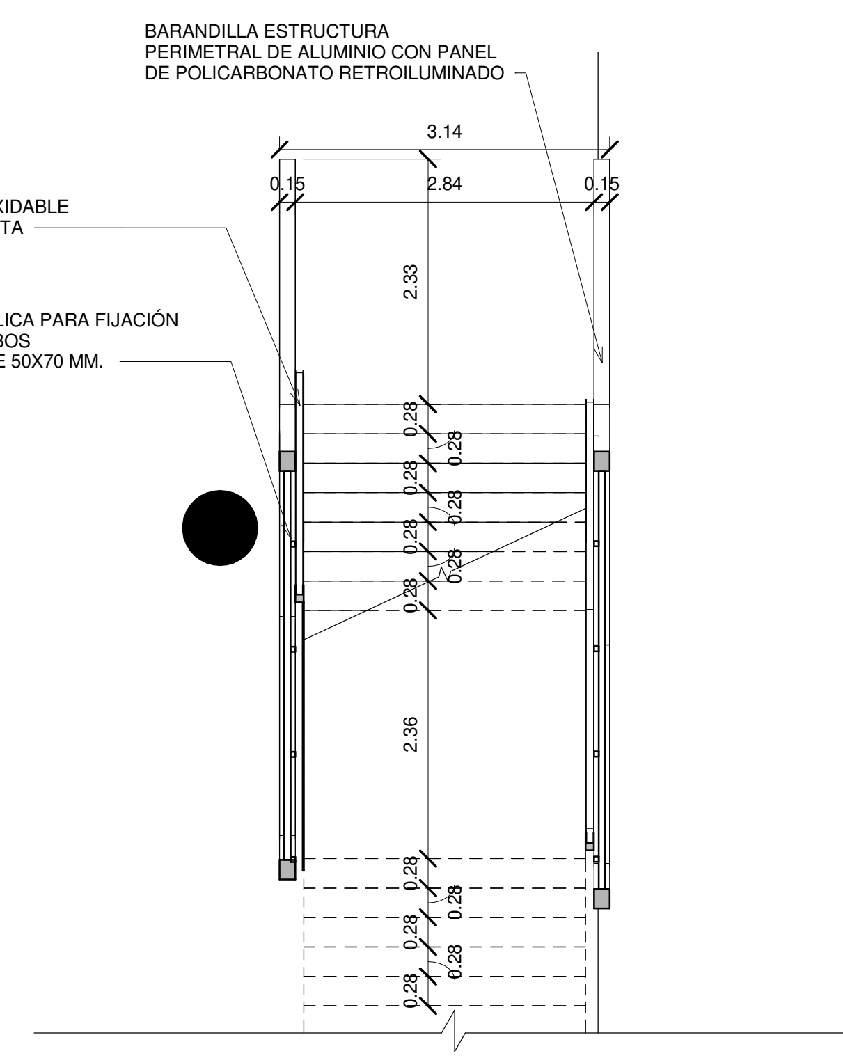
1 A-01 DETALLE EN PLANTA ESCALERA EXTERIOR 1 : 50
