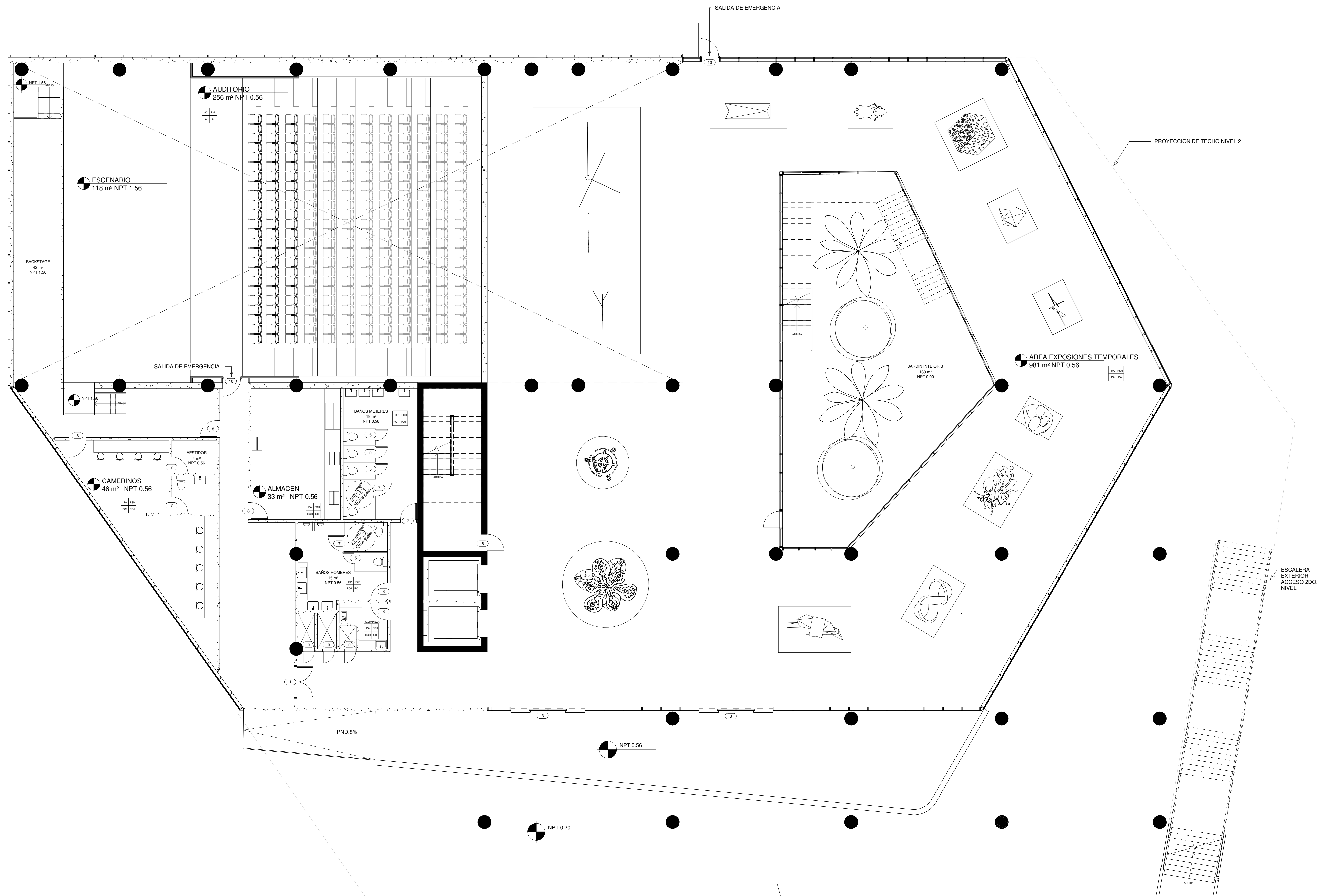
1 A-07 PLANTA ARQUITECTÓNICA AMUEBLADA NIVEL 1- ZONA C 1 : 100
