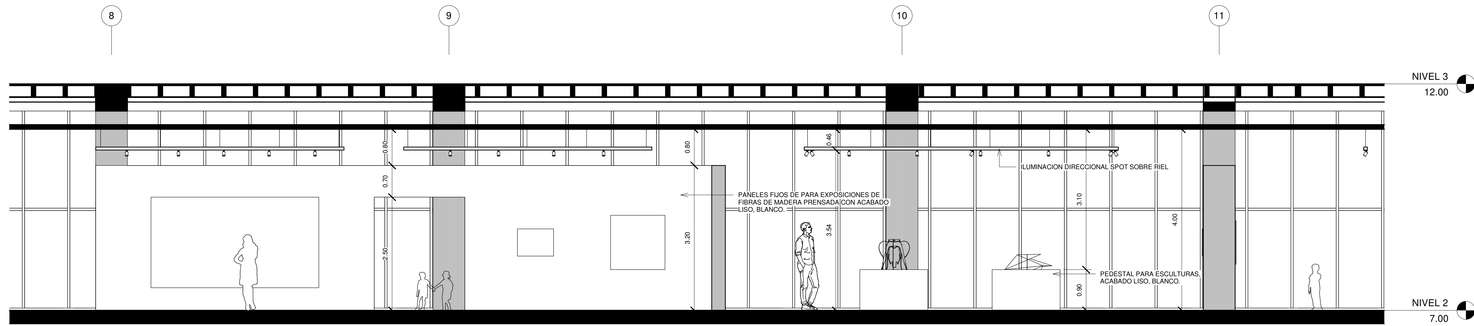
1 SECCION 1 AREA DE EXPOSICIONES PERMANENTES A 1 : 50
