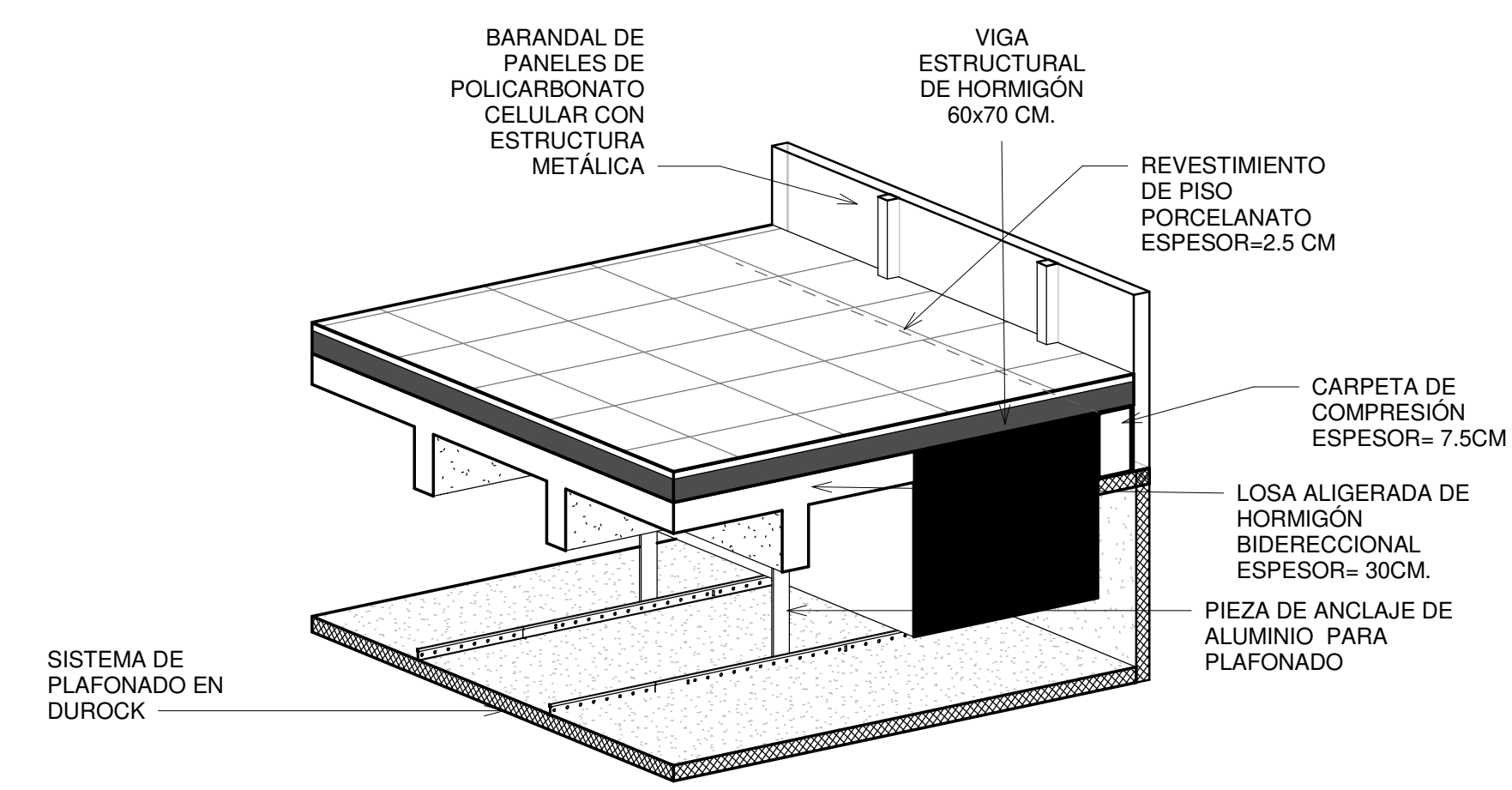
5 DETALLE ENTREPISO 1:20
