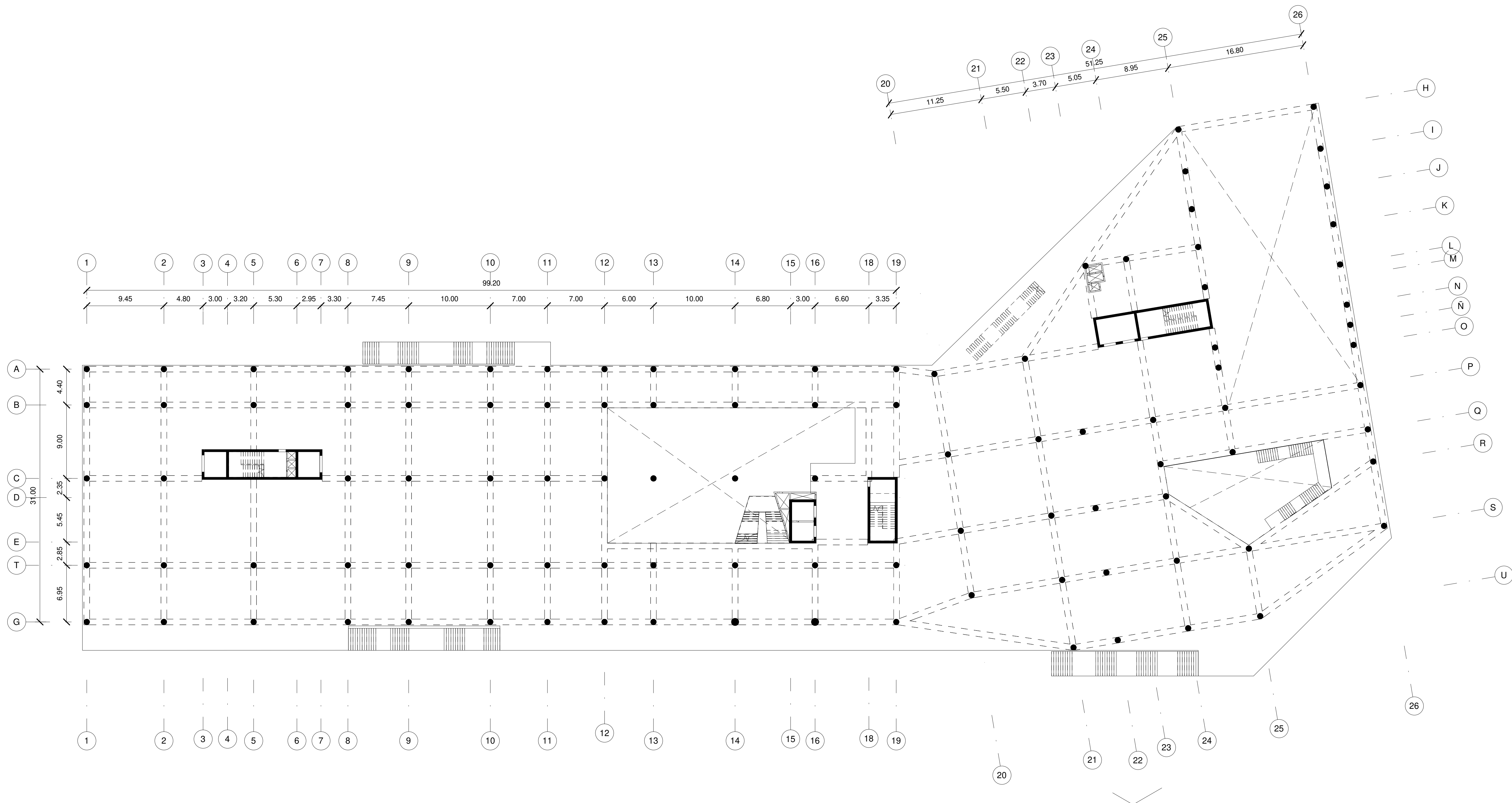
1 PLANTA ESTRUCTURAL NIVEL 2 1 : 250
