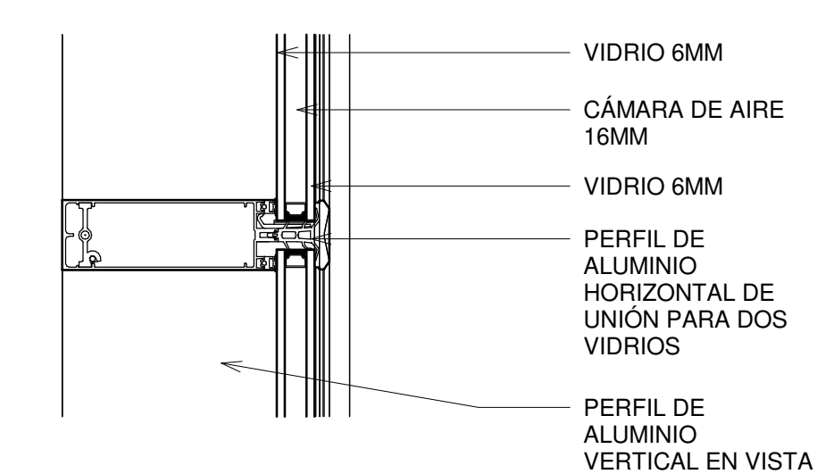
4 DETALLE UNION MURO CORTINA 1:5
