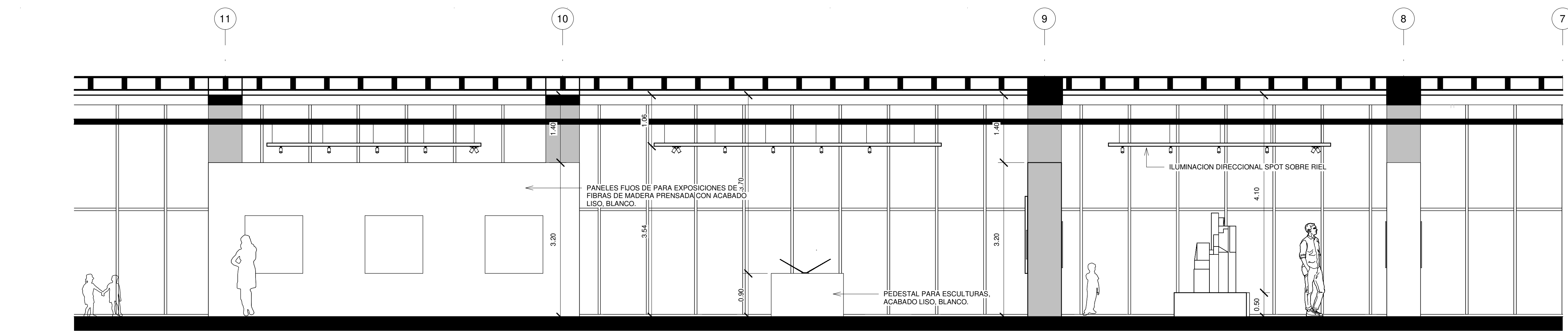
4 SECCION 3 AREA DE EXPOSICIONES PERMANENTES A 1 : 50
