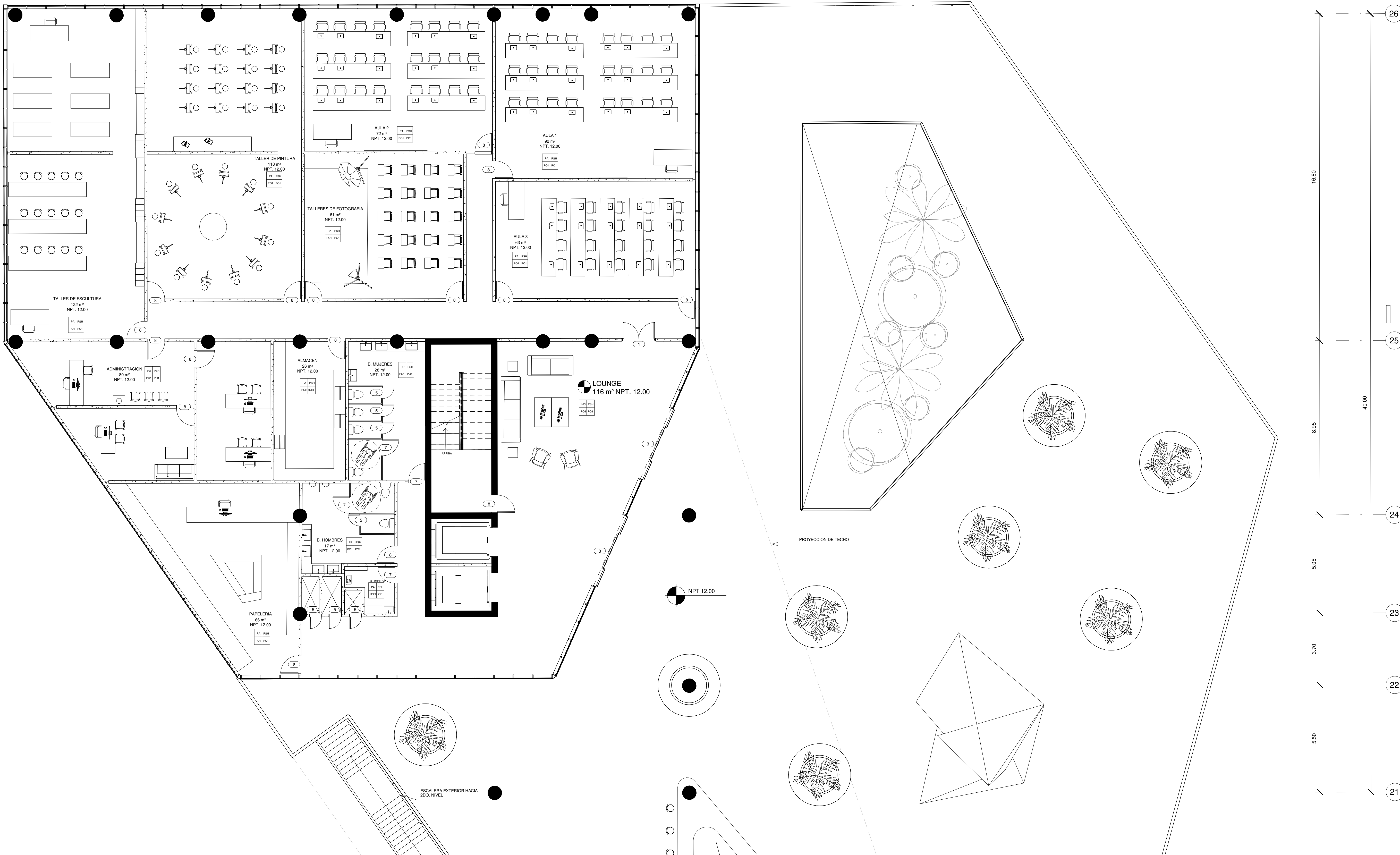
1 A-23 PLANTA ARQUITECTÓNICA AMUEBLADA NIVEL 3 - ZONA C 1 : 100
