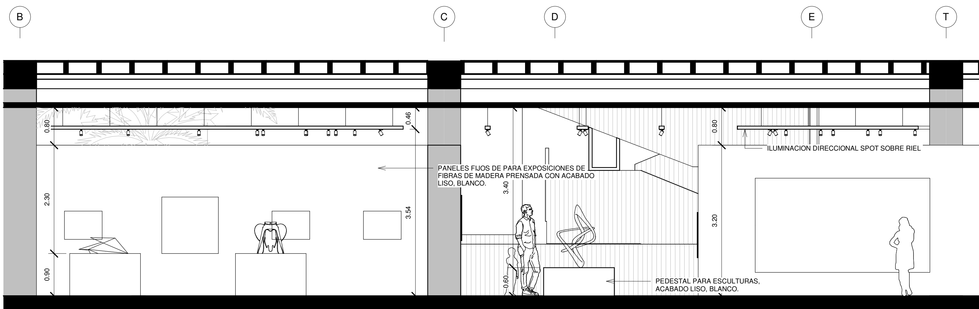
4 SECCION 3 AREA DE EXPOSICIONES PERMANENTES A 1 : 50
