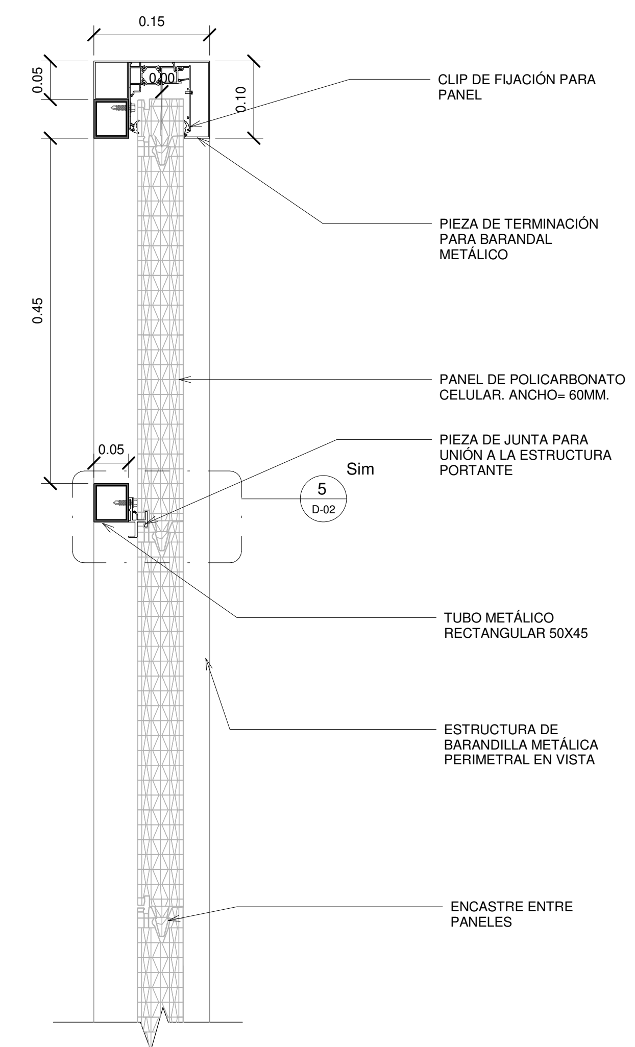
4 Detalle Unión entre paneles de policarbonato 1 : 5
