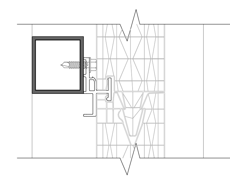
5 DETALLE ANLAJE 1 : 2
