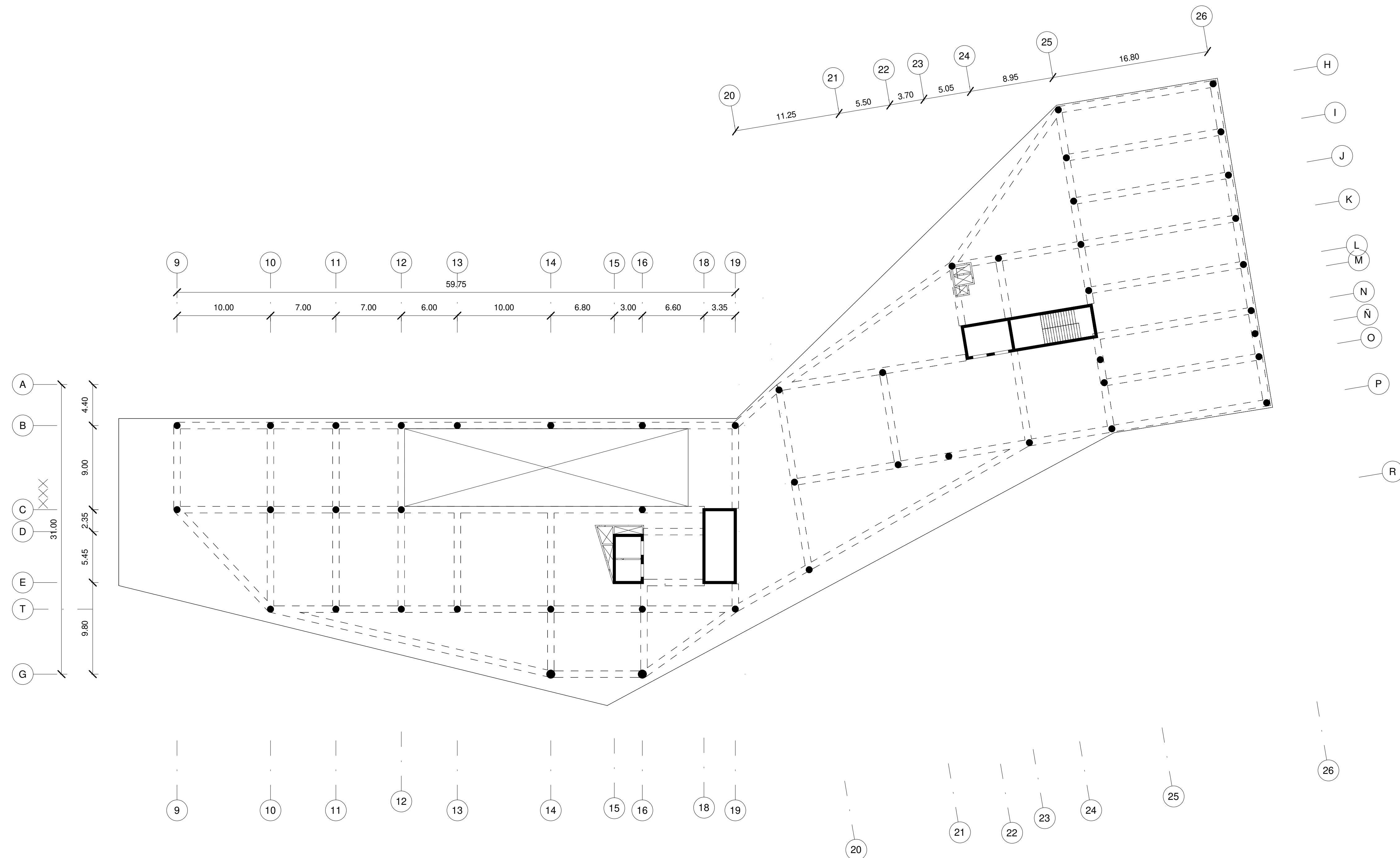
1 PLANTA ESTRUCTURAL NIVEL 4 1 : 250
