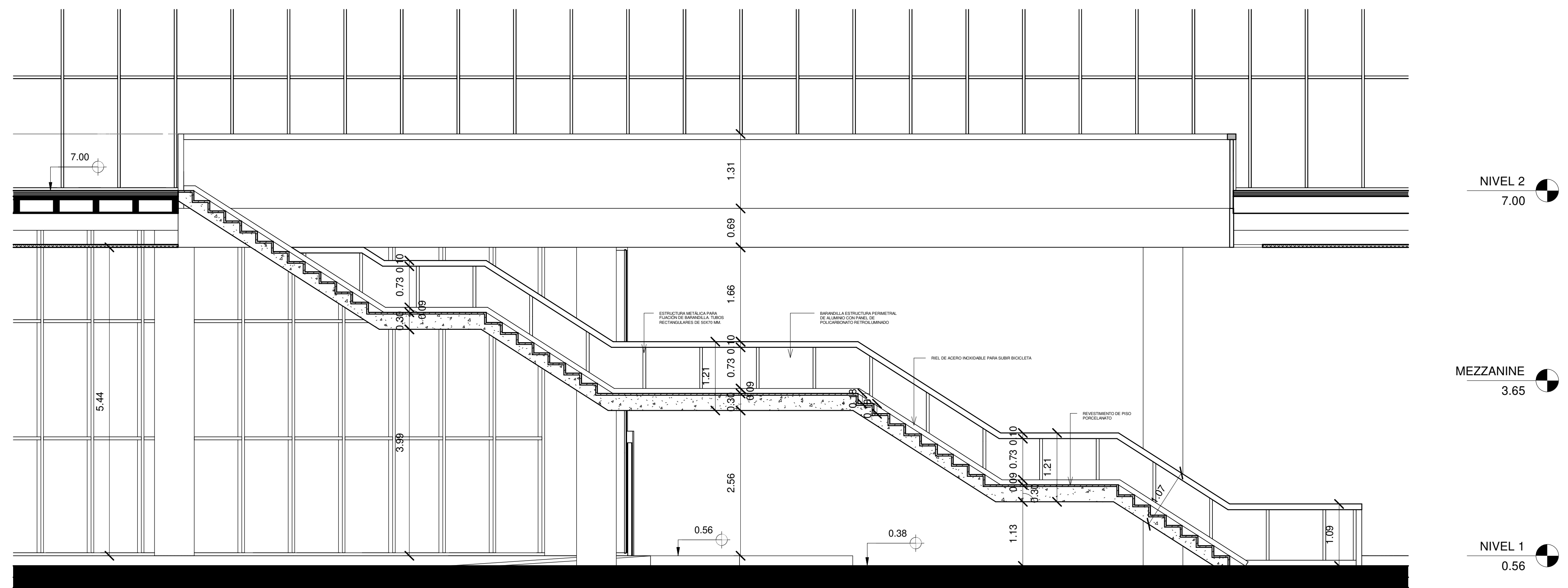
2 DETALLE DE ESCALERA SECCION 1 : 50
