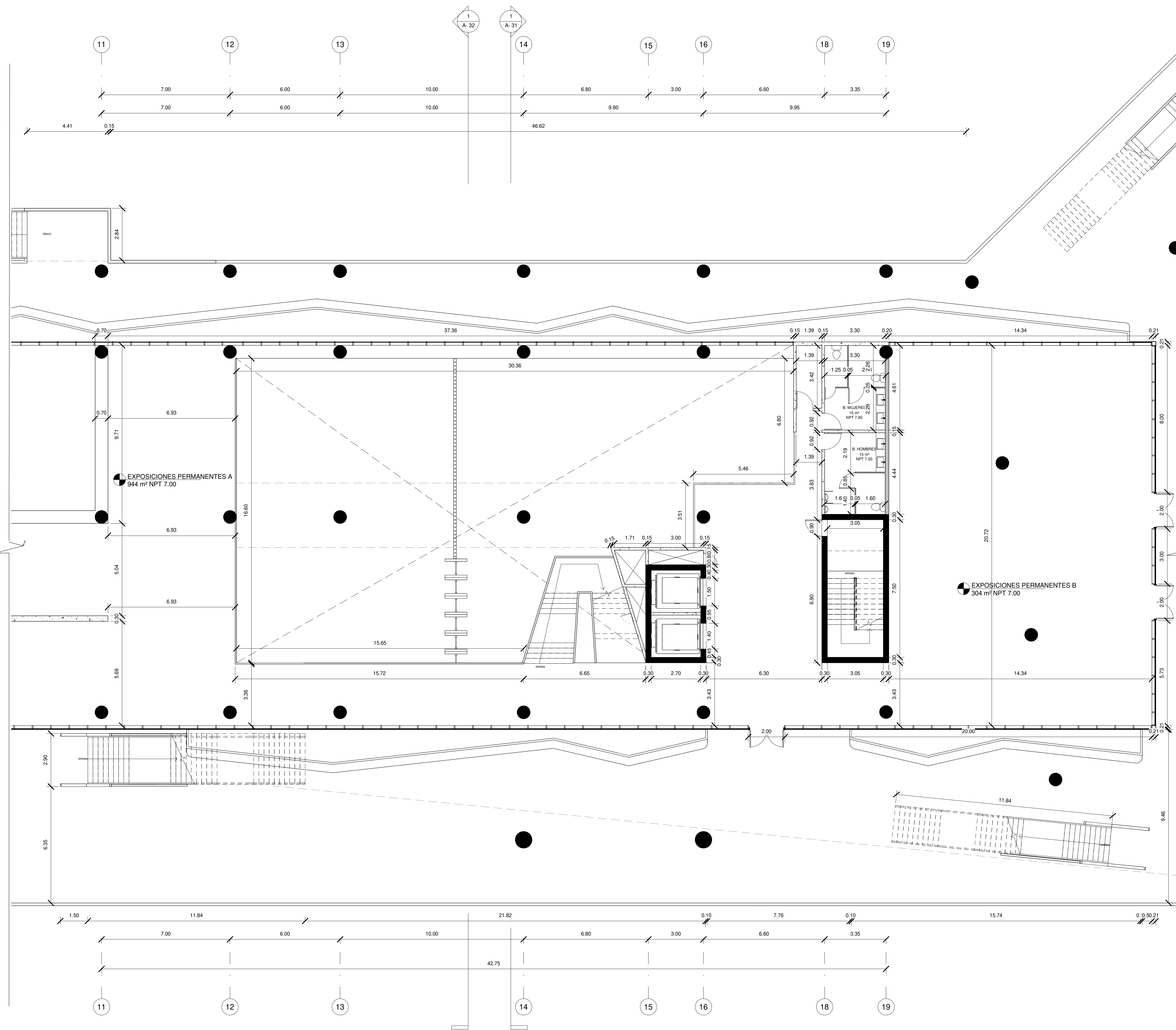
1 A-15 PLANTA ARQUITECTÓNICA DIMENSIONADA NIVEL 2 - ZONA B 1 : 100
