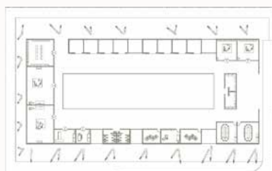
Planta Veterinaria, Servicios, Admin./Gimnasio
